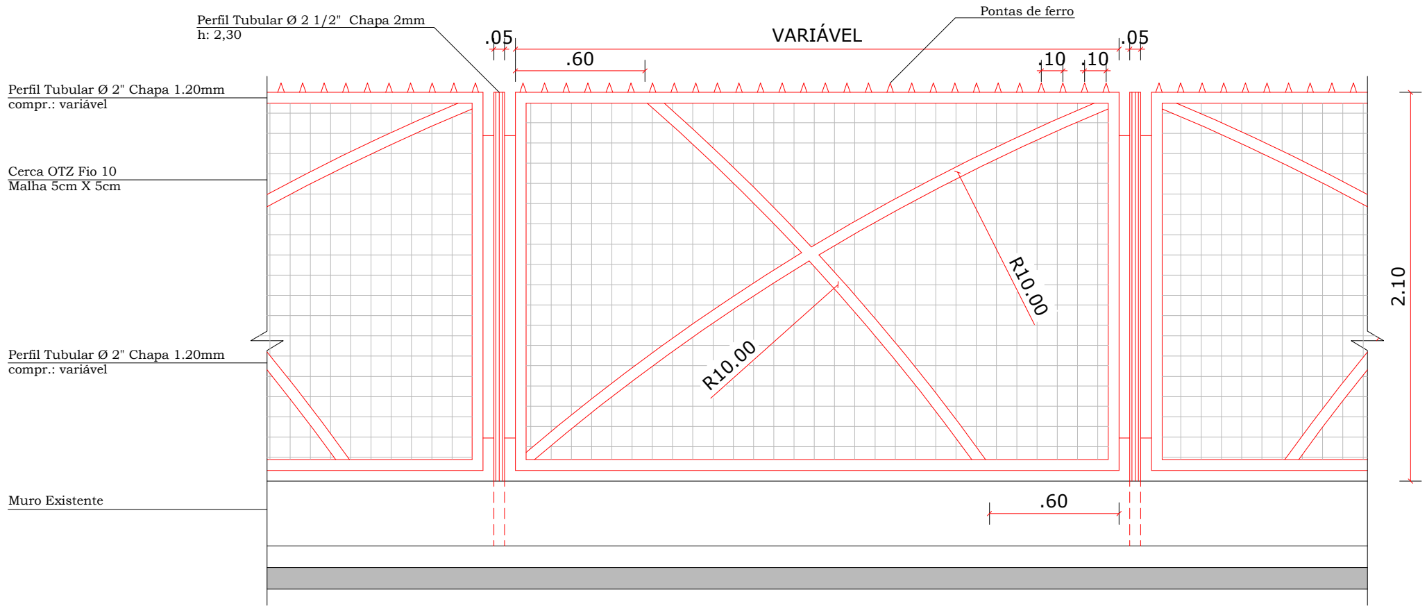
DETALHE CERCADO SOBRE MURO ESC.....1/25
