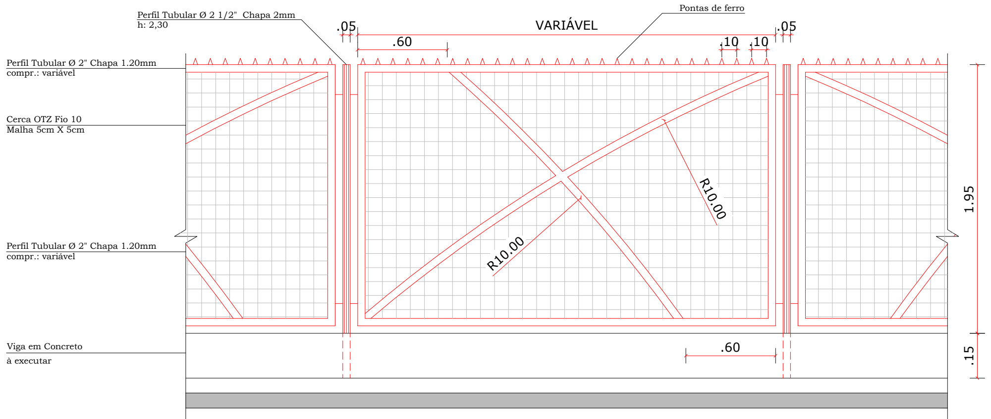
DETALHE CERCADO COM VIGA ESC.....1/25
