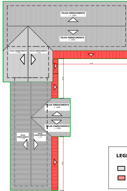
PLANTA DE COBERTURA Sem escala
