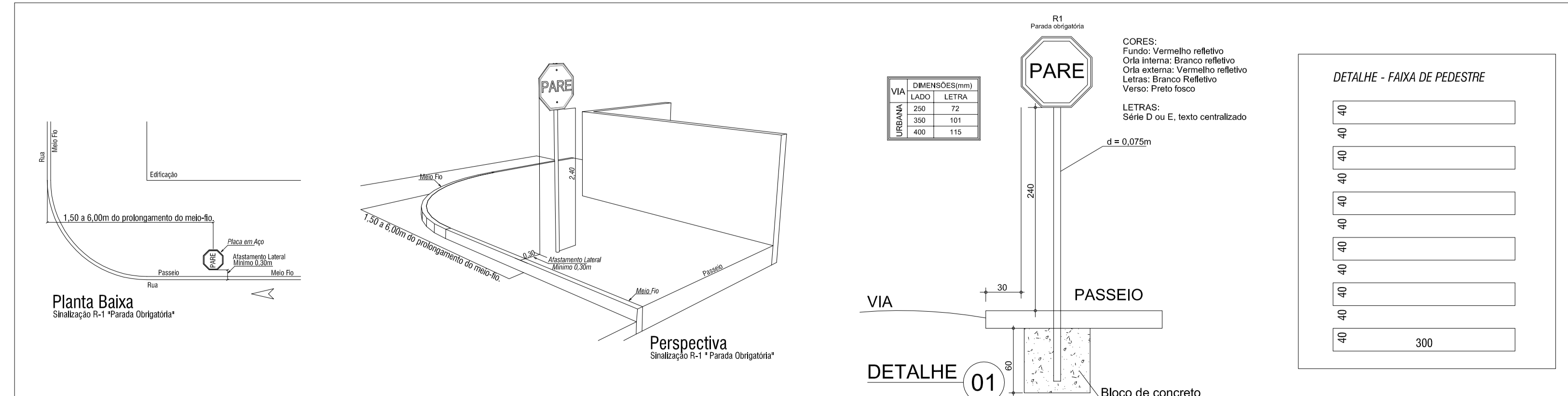
DETALHAMENTO SINALIZAÇÃO
