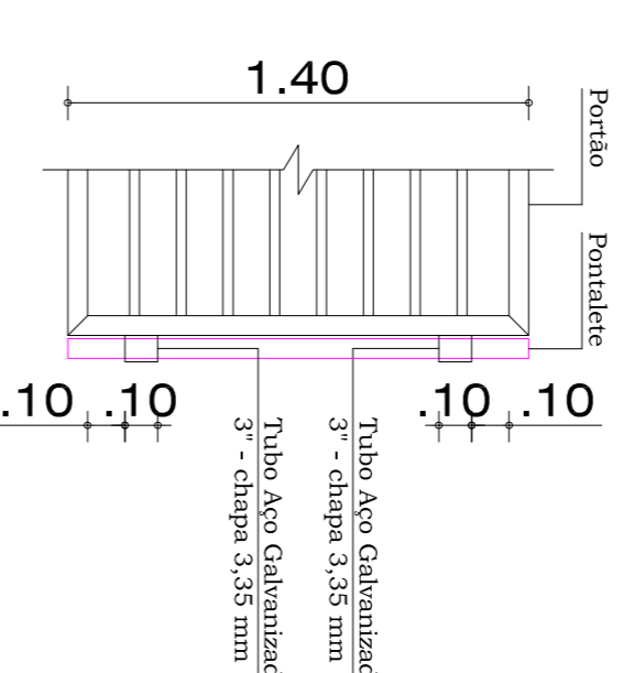
Detalhe Fixação dos Portões ESC.....1/50
