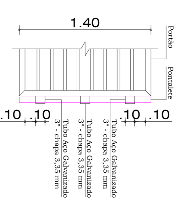
Detalhe Fixação dos Portões ESC.....1/50
