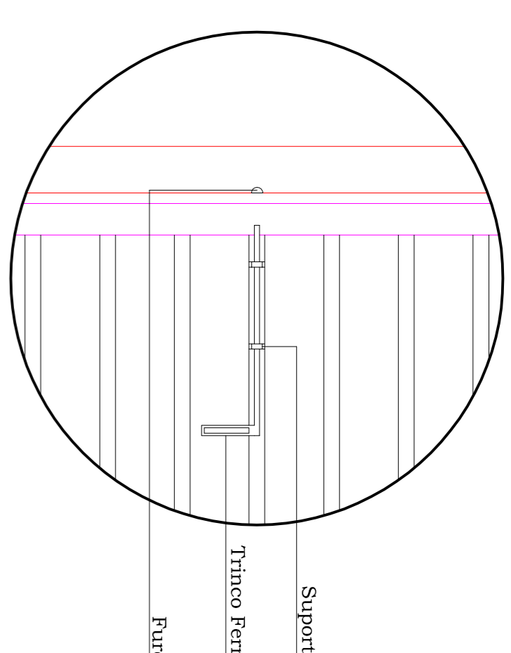
Detalhe Fechamento Portões ESC.....1/10
